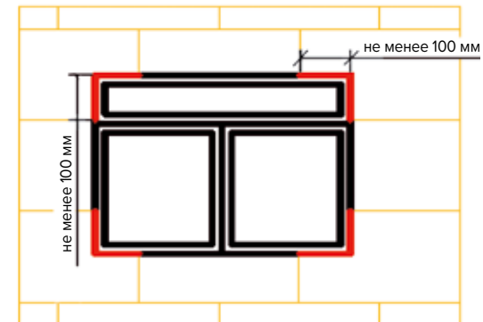
Расположение утеплителя в углах проемов
